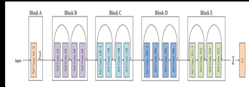
딥러닝 기반
